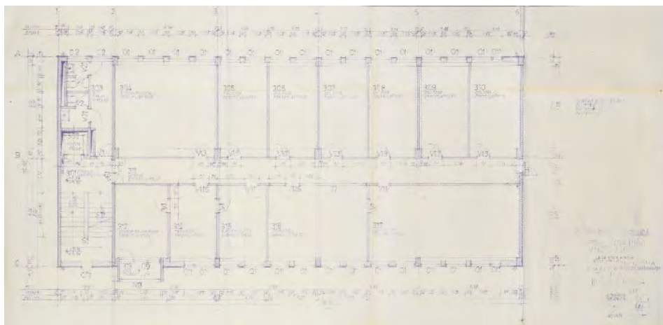
Tloris delovnih prostorov arhiva, avtor Roni Nemec, 1986 (SI_PANG/0337 Pokrajinski arhiv v Novi Gorici, Poslovna hiša PA – LB v Novi Gorici, gradbeno-obrtniška dela, načrti).
