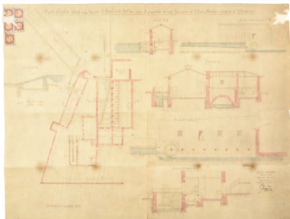
Načrt mlina v Peklu pri Braniku, 1927 (SI_PANG/0021 Tehnični urad Gorica, t. e. 13, p. e. 304).
